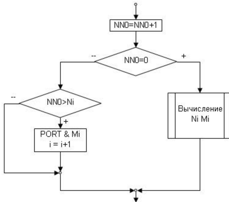
Рисунок 1. Экономичный алгоритм формирования ШИМ сигнала
